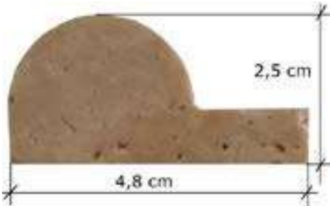
GH-COR-120 GH-COR-121 GH-COR-122 GH-COR-123 GH-COR-124 Travertin LIGHT 4,8 x 2,5 x30,5 cm Travertin NOÇE4,8 x 2,5 x30,5 cm Travertin SILVER 4,8 x 2,5 x30,5 cm Travertin AUTUMN 4,8 x 2,5 x30,5 cm Travertin ROSE 4,8 x 2,5 x30,5 cm
